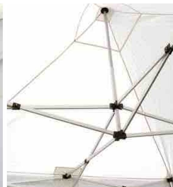
Art. GAZ 110 Gazebo quadrato 3 x 3 m. Mercato Struttura in alluminio esagonale 40 mm. con traliccio centrale Poliestere 300 gr. bianco impermeabilizzato e interno in PVC con sacca per il trasporto
